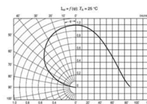
CARACTÉRISTIQUE DE RADIATION
